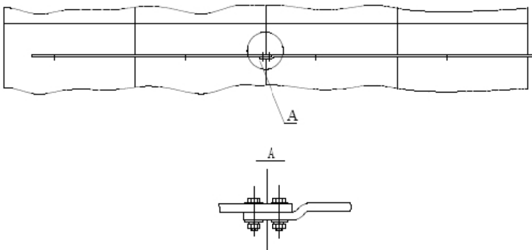
Схема монтажа сборных шин камер КСО (вид сверху)
