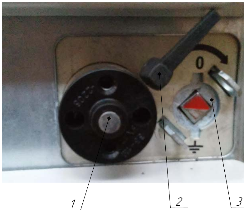
Рисунок 3 - Выключатель заземления
