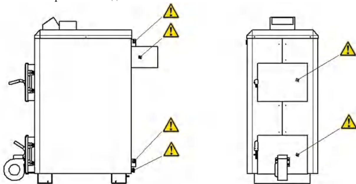
Рисунок Ж.1 Схема горячих поверхностей
