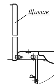
Рисунок 7 – Крепление щитка
