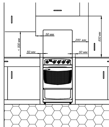
Рисунок 6 – Схема установки плиты
