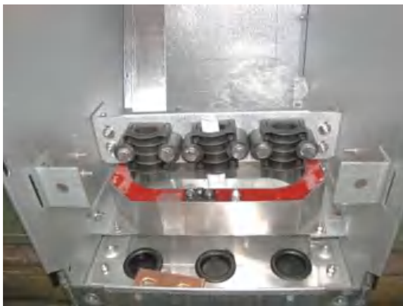
Внешний вид трансформаторов тока
