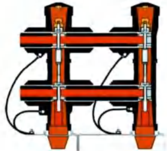
Рисунок 5 - Сборные шины на 1600 А, 2000 А, 2500 А
