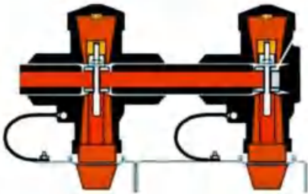
Рисунок 4 - Сборные шины на 1250 А
