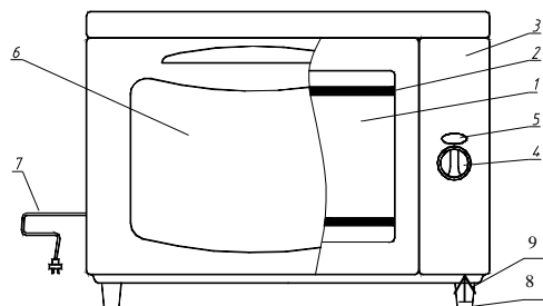
Приложение Б (обязательное) Устройство электрошкафа
