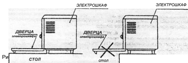
Приложение А (обязательное) Установка электрошкафа на столе
